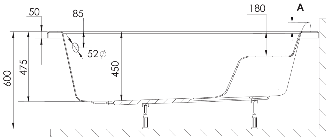
ŘEZ A-A
